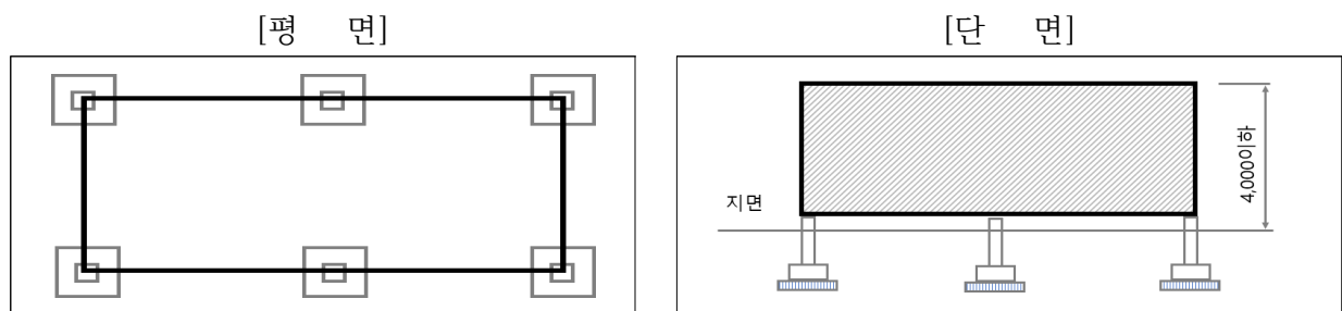
<독립기초 형식 예시도>
